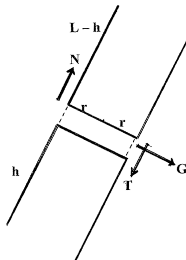
Figur 3. Snit vilkårligt sted i faldende skorsten.
