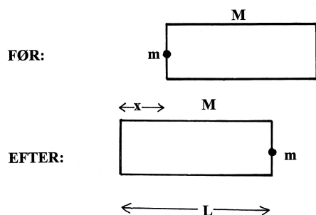
Figur 3. Einsteins tankeeksperiment.
