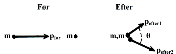
Figur 2. Uelastisk spredning af en puck på en anden puck.
