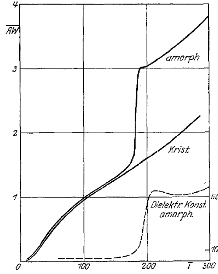
Fig. 2. Atomwärmern des Glycerins. Von 300 bis 70° abs. nach Simon (l. c.) und Gibson und Giaugue, unterhalb 70° nach dieser Arbeit.
