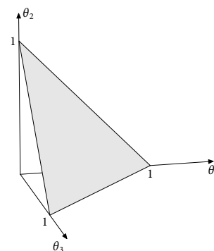
Sandsynlighedssimplexet i det tredimensionale rum, dvs. mængden af ikke-negative tripler (\theta_1, \theta_2, \theta_3) med \theta_1 + \theta_2 + \theta_3 = 1 .
