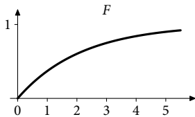
Tæthedsfunktion og fordelingsfunktion for eksponentialfordelingen med \beta = 2.163 .
