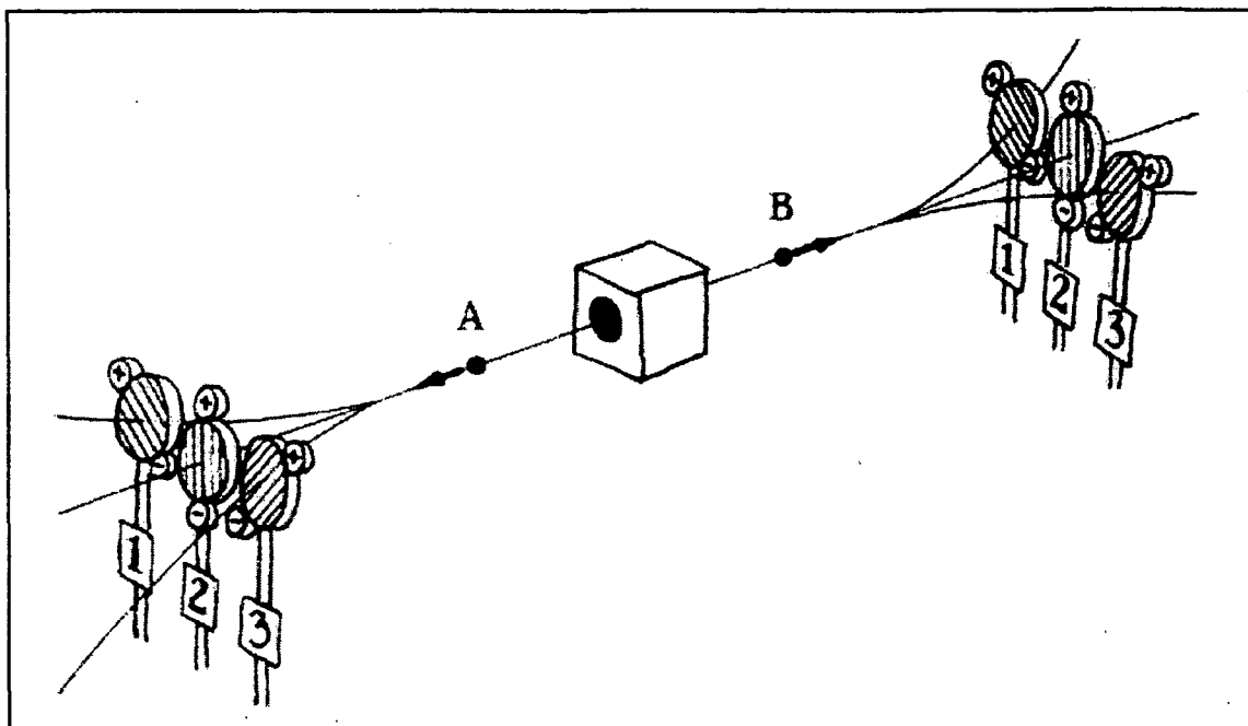
Figur 14.1. Aspect's forsøg. Et par af partikler med modsatte egenskaber (+ og -) dannes i kassen midt i billedet og bevæger sig ud til hver sin side. For hver af dem kan Aspect vælge, hvilket af de tre måleapparater partiklen skal gå igennem, og hermed vælge, i hvilken retning egenskaben skal måles.
