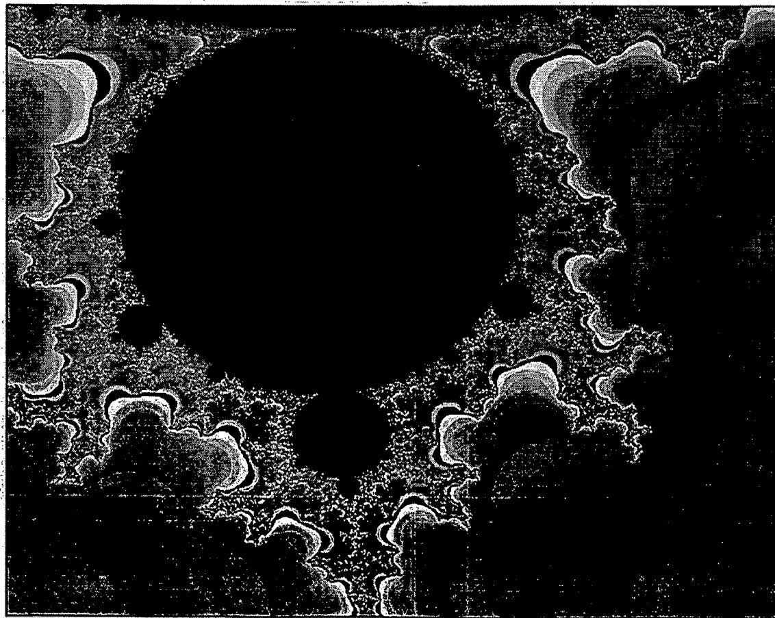
Figur 16.4a. Udsnit af Mandelbrotmængdens rand, repræsenteret ved farve/gråtone skala.
