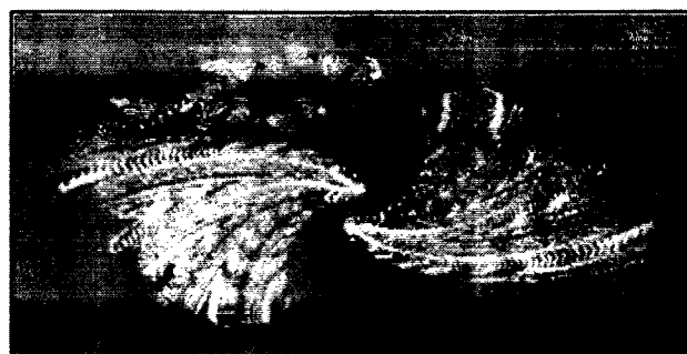
Figur 16.4d. Udsnit af Juliamængden, der er komplementær til Mandelbrotmængden.
