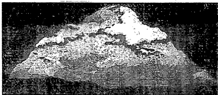
Figur 16.3. Fraktalt bjerglandskab med tilfældig højdevalg for hver ny underopdeling af trekantmønstreet.
